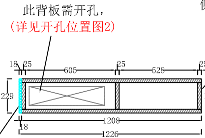
剖面图C-C
