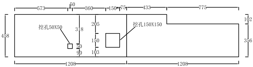
盖板（平面图）
