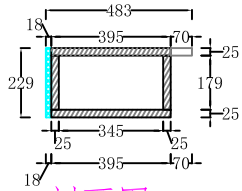
剖面图B-B
