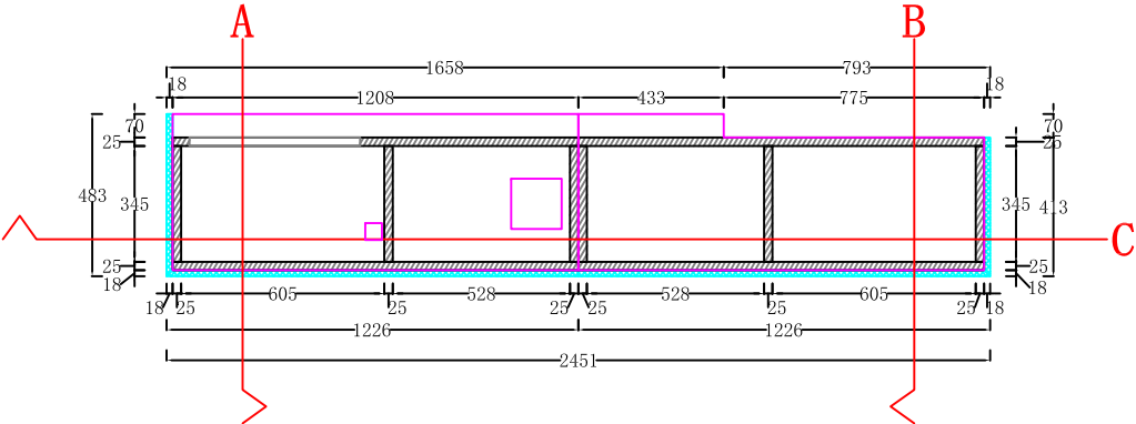
分成2个独立箱体-俯视图
