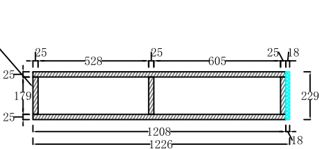
剖面图C-C
