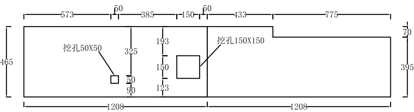
盖板（平面图）
